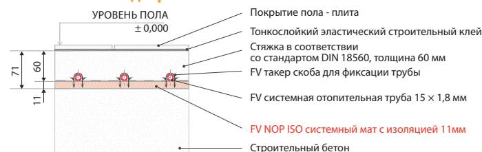
Рисунок 16: Рекомендуемый состав пола над отопляемыми помещениями в соответствии со стандартом ČSN EN 1264 термостойкость изоляции R=0,75 м² К/В
