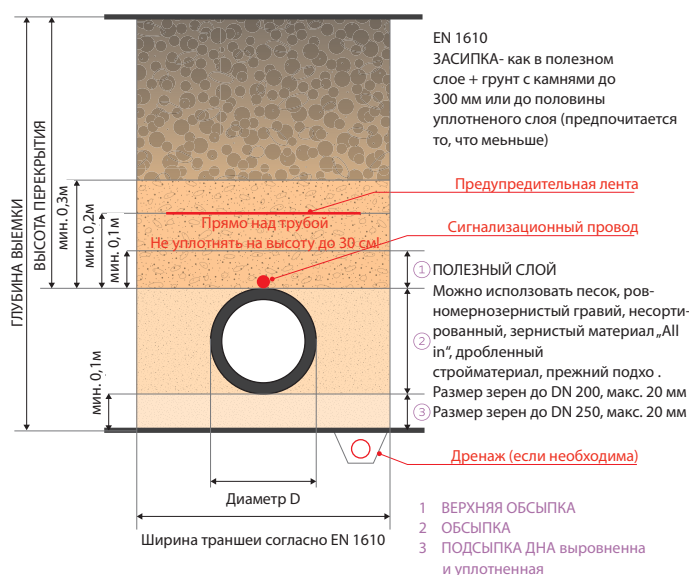
Схема укладки труб FV HDPE 100 в транше
