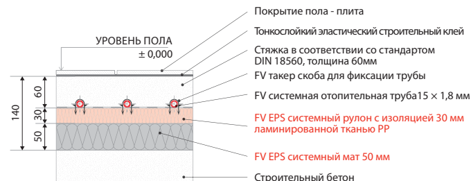
Рисунок 18: Рекомендуемый состав пола над открытым пространством в соответствии со стандартом ČSN EN 1264 термостойкость изоляции R=2,00 м² К/В
