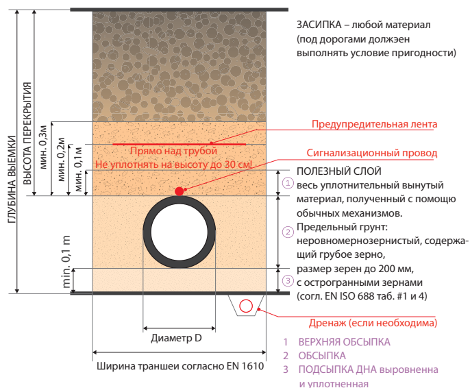
Схема укладки труб FV HDPE 100 RC в транше
