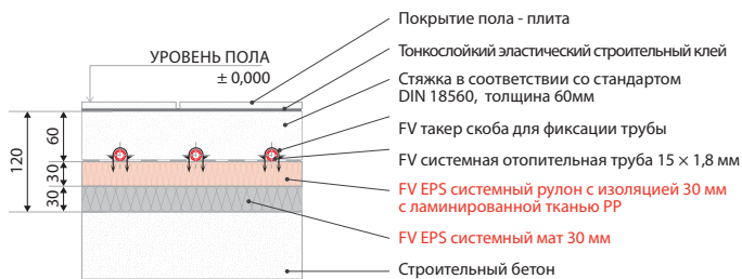
Рисунок 17: Рекомендуемый состав пола в подвальных и малоотпливаемых помещениях в соответствии со стандартом ČSN EN 1264 термостойкость изоляции R=1,25 м² К/В
